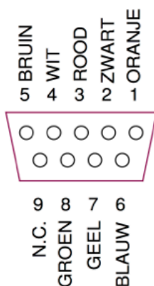
ACHERTERZIJDE D9 MALE CONN
